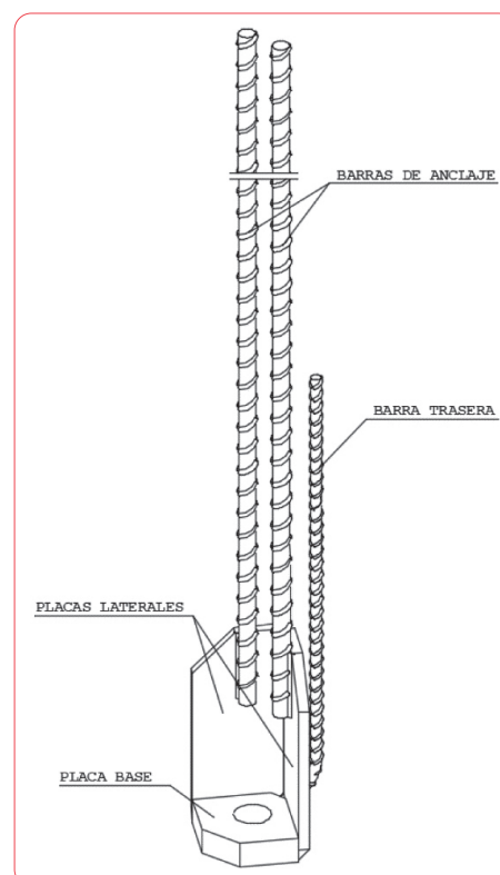
Imagen 7: Componentes PDP
