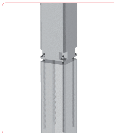
Imagen 5: Unión pilar-pilar
