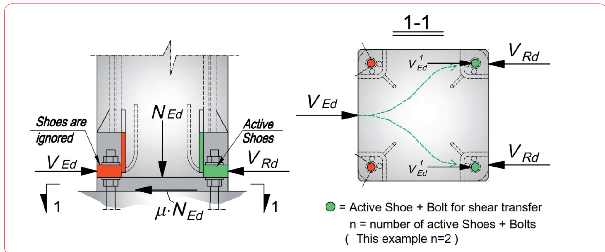
Imagen 9: Solo los pies de pilar en el lado derecho se consideran activos ante cortante
