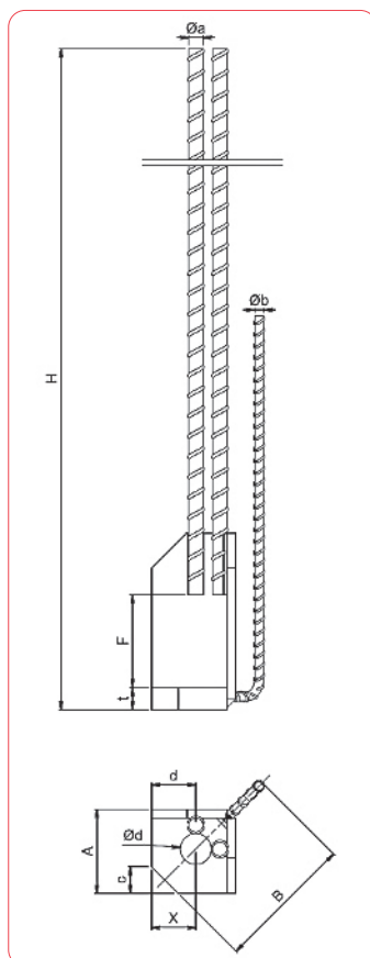
Imagen 6: Dimensiones PDP
